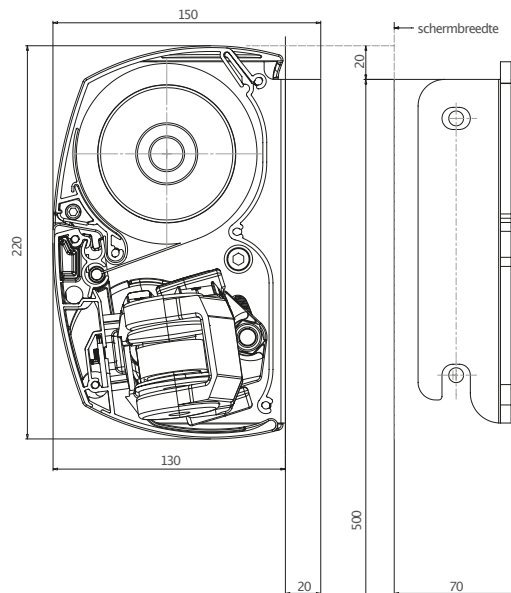
Fiora Compactverlengde montage
